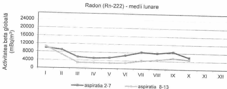
Figura 21. Activitatea calculată a Radonului
