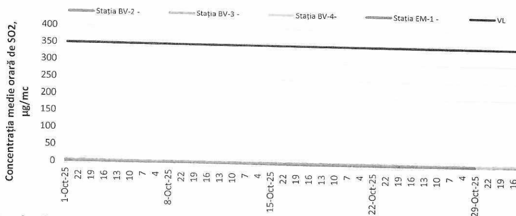
Figura 2. Evoluția mediilor orare de SO 2 în luna octombrie 2025
