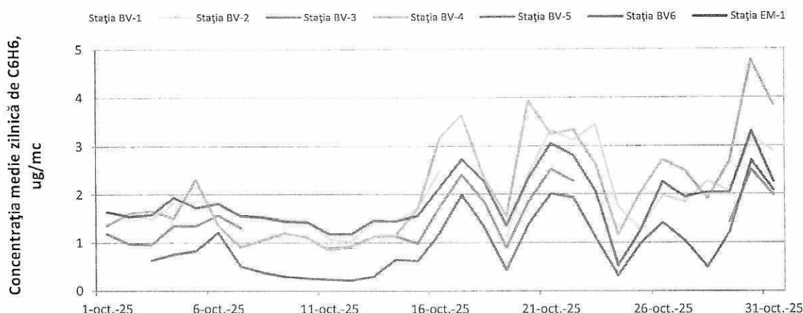
Figura 7. Evoluția concentrațiilor medii zilnice de benzen în luna octombrie 2025
