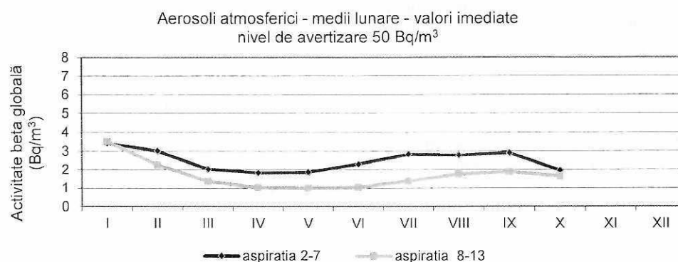
Figura 20. Activitatea beta globală pentru aerosoli atmosferici
