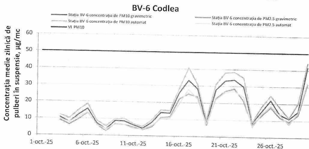
Figura 12. Evoluția concentrațiilor medii zilnice de PM10 gravimetric și automat și PM2,5 gravimetric și automat în stația de fond urban BV-6 în luna octombrie 2025
