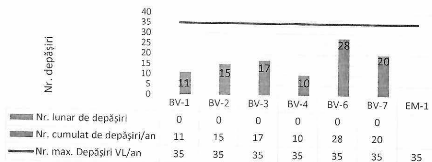
Figura 9. Numărul lunar și cumulat de depășiri ale valorii limită zilnice la PM10
