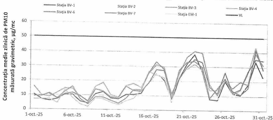
Figura 8. Evoluția concentrațiilor medii zilnice de PM10 (gravimetric) în luna octombrie 2025
