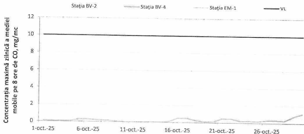
Figura 4. Concentrația maximă a mediei mobile pe 8 ore de CO în luna octombrie 2025
