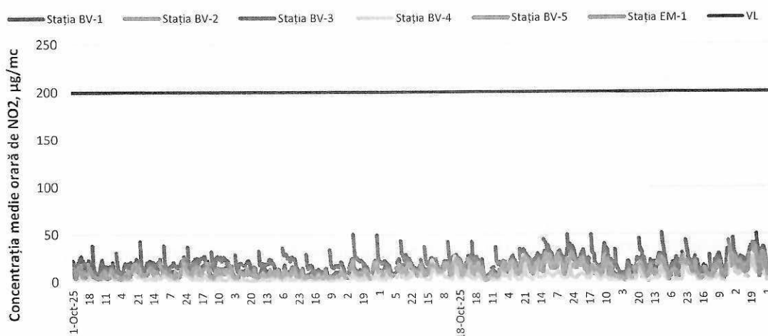
Figura 3. Concentrații medii orare de NO 2 în luna octombrie 2025
