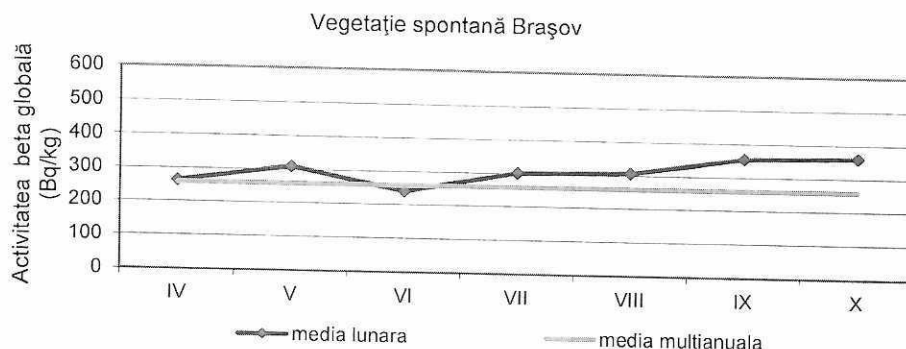
Fig. 28. Activitatea beta globală la 5 zile pentru solul necultivat
