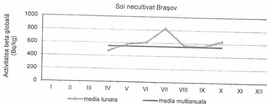
Fig. 27. Activitatea beta globală la 5 zile pentru solul necultivat
