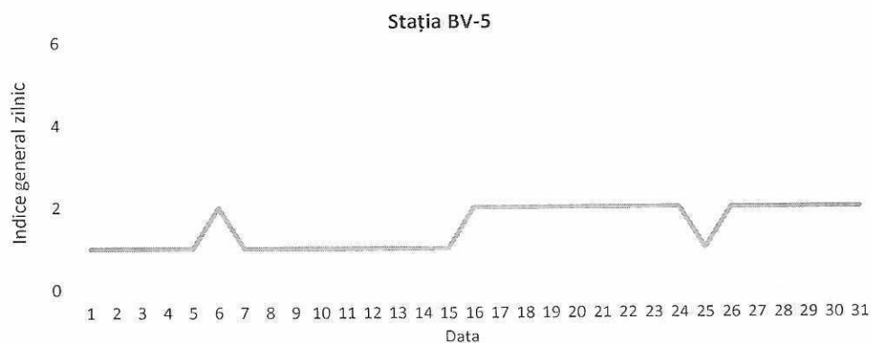
Figura 17. Evoluția indicelui general de calitate a aerului din stația BV-5
