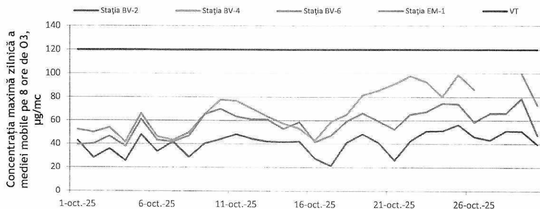
Figura 5. Evoluția concentrațiilor maximelor zilnice ale mediilor mobile pe 8 ore de O 3 în luna octombrie 2025
