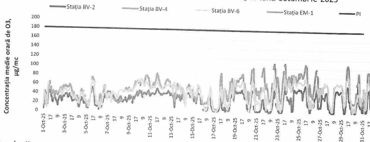
Figura 6. Evoluția concentrațiilor medii orare de O 3 în luna octombrie 2025
