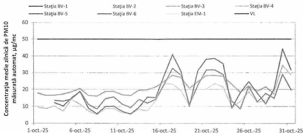
Figura 10. Evoluția concentrațiilor medii zilnice de PM 10 automat în luna octombrie 2025
